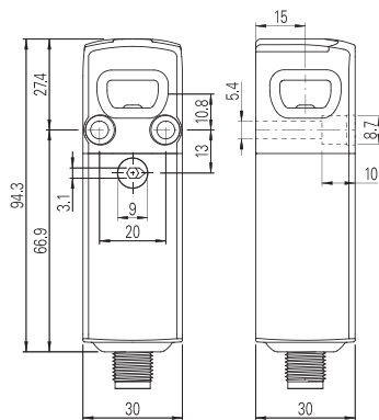
Dispositivo NX ●●●AZ●SMK
