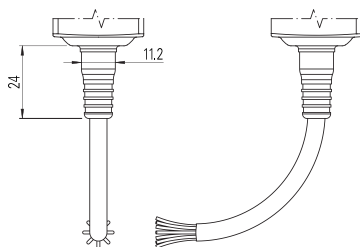
Con cable axial
