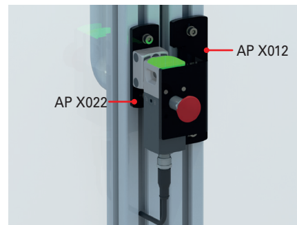
Drehtüren, mit Befestigung des Schalters auf der Innenseite der Tür.
