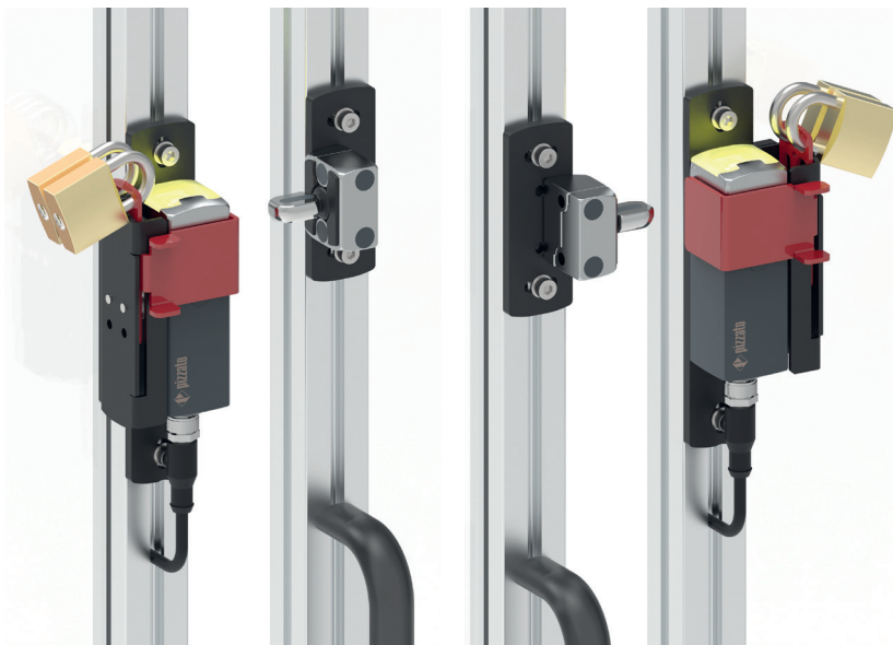
Konfiguration für Schutzvorrichtung mit Dreh- und Schiebetür, nach rechts öffnend. LK X1S001
