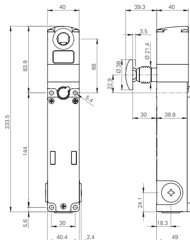
Schalter NG 2D7E••1A Funktionsprinzip E, mit Fluchtentsperrungstaster, ohne Betätiger
