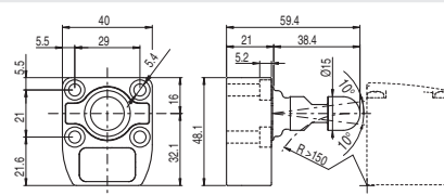
Betätiger VN NG-F3•
