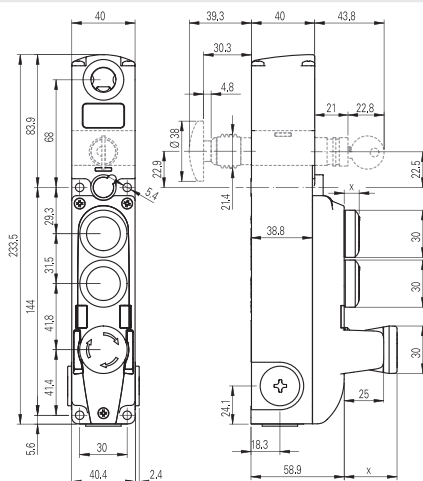
Schalter NG 2D●●●●● mit integrierten Befehlsgebern
