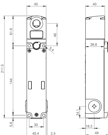
Schalter NG 2D1E••1A Funktionsprinzip E, ohne Betätiger
