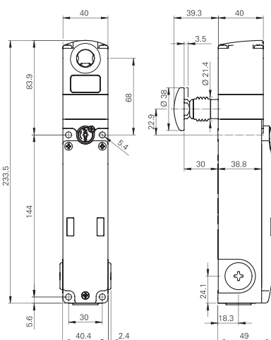
Schalter NG 2D7D••1A Funktionsprinzip D, mit Fluchtentsperrungstaster, ohne Betätiger
