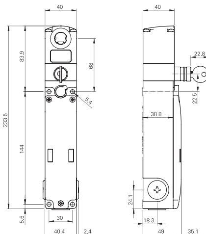
Schalter NG 2D5D••1A Funktionsprinzip D, mit Hilfsentsperrung mit Schloss, ohne Betätiger
