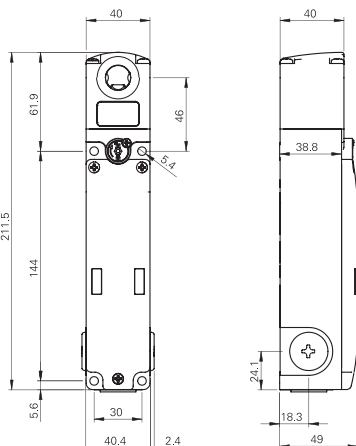
Schalter NG 2D1D••1A Funktionsprinzip D, mit verplombbarer Hilfsentsperrung, ohne Betätiger
