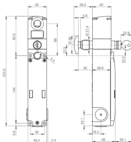
Schalter NG 2D6D••1A Funktionsprinzip D, mit Hilfsentsperrung mit Schloss und Fluchtentsperrungstaster, ohne Betätiger
