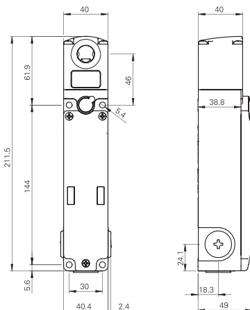
Interruttore NG 2D7D●●1 A
