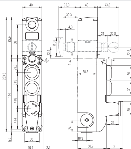
Interruttore NG 2D●●●●●● con dispositivi di comando integrati
