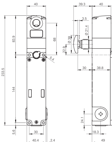
Azionatore VN NG-F3•
