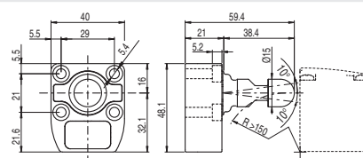
Azionatore VN NG-F3•
