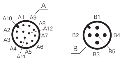
Connecteur M12 double à 12 pôles
