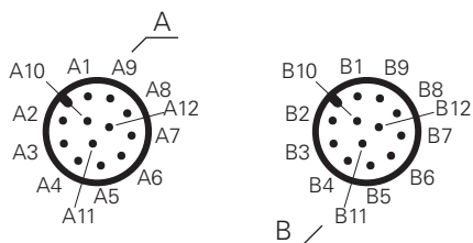
Connecteur M12 double à 12 pôles
