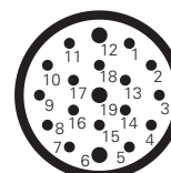
M23-Steckverbinder, 19-polig
