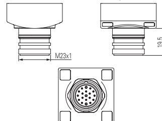
M23-Steckverbinder, axial
