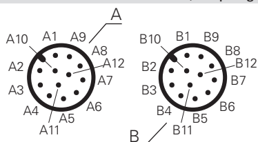
Zwei M12-Steckverbinder, 12-polig
