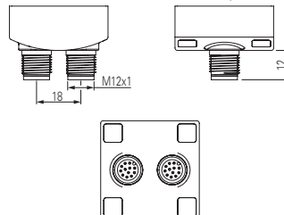
Zwei M12-Steckverbinder, axial
