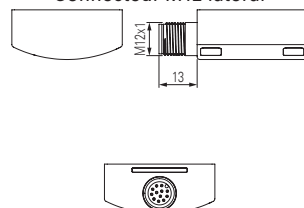
Connecteur M12 latéral
