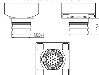
Connecteur M23 axial
