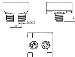
Connecteur M12 double axial
