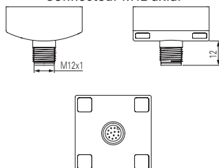
Connecteur M12 axial
