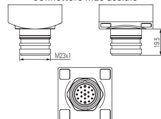
Connettore M23 assiale
