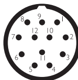
Connettore M23 a 12 poli
