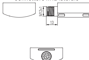
Connettore M12 laterale
