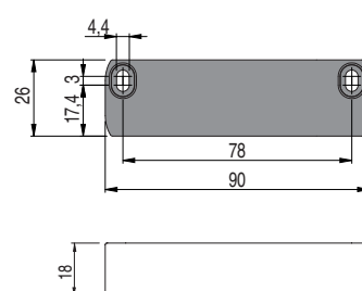
Actuador SM E•T
