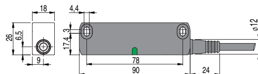
Sensor ST H••••N• mit Kabel
