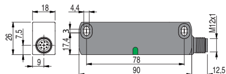
Sensor ST H••••M• mit M12-Steckverbinder
