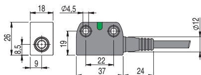
Sensor ST G••••N• mit Kabel
