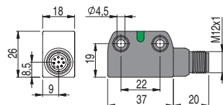
Sensor ST G••••M• mit M12-Steckverbinder
