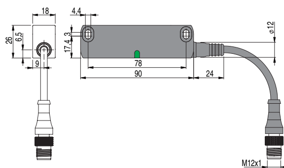
Sensor ST H••••M0.2 Kabel und M12-Steckverbinder
