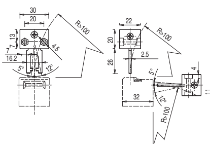
Actuator VF KEYF8
