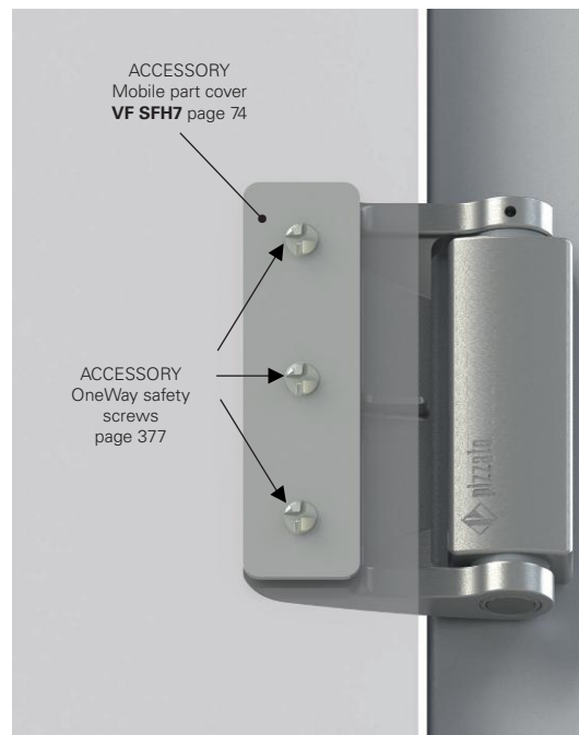
Open door
